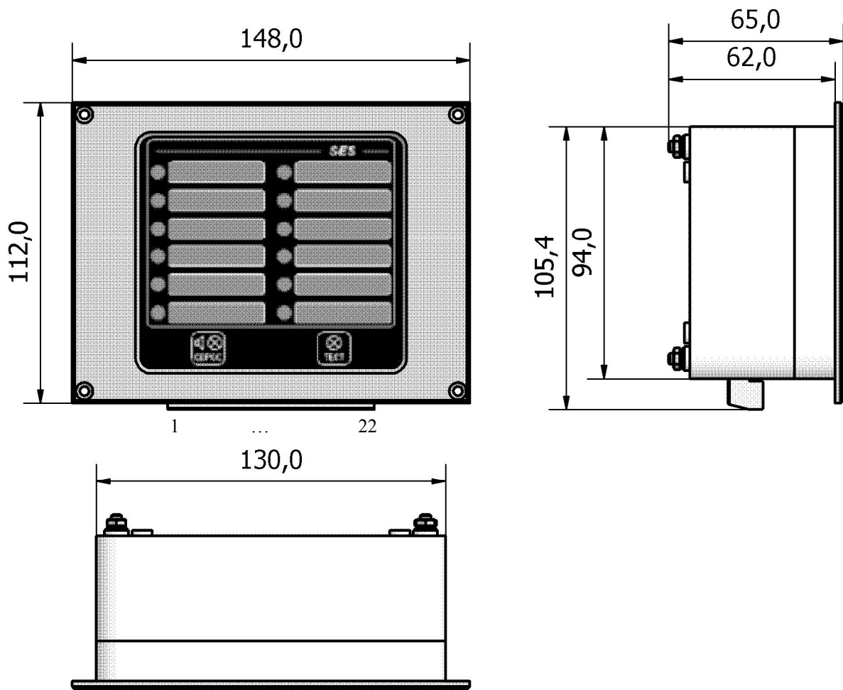
Блок сигнализации «SES». Габаритный чертеж
